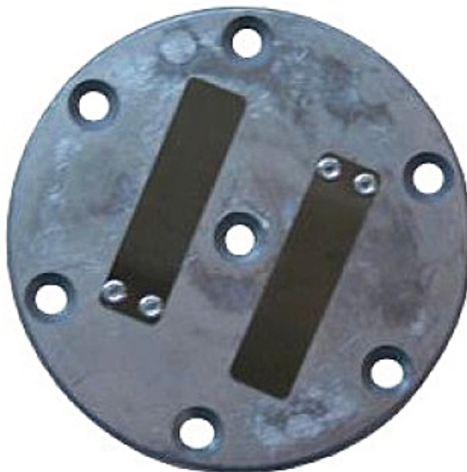
Płytką zaworowa sprężarki dolna
