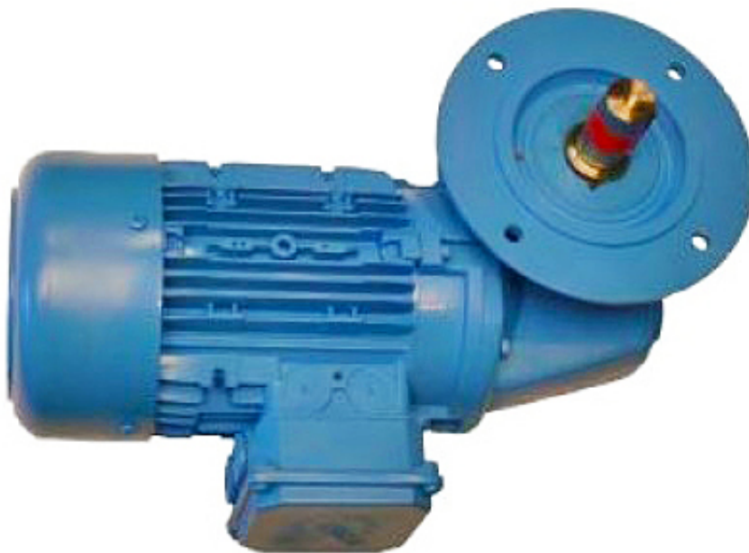
Motoreduktor 1,1 kW kątowny
